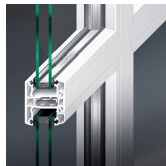
Glasteilende Sprosse
