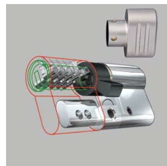
Sicherheitsprofilzylinder 1 K4000
