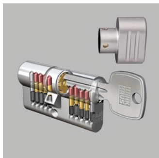
Profilzylinder 4 W XR 51
