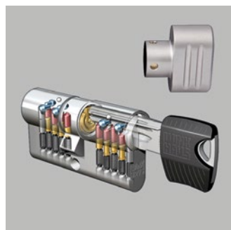
Profilzylinder 5 RPE 51
