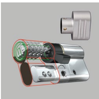
Sicherheitsprofilzylinder 2 K4000 mit Anbohrschutz
