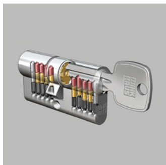
Profilzylinder 4 W XR 51 ohne Knauf
