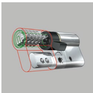
Sicherheitsprofilzylinder 1 K4000 ohne Knauf
