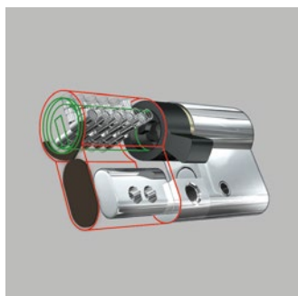
Sicherheitsprofilzylinder 2 K4000 ohne Knauf mit Anbohrschutz
