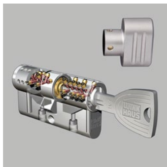
Sicherheitsprofilzylinder 6 W XT51
