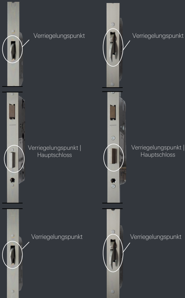
Schwenkhakenschluss manuell
